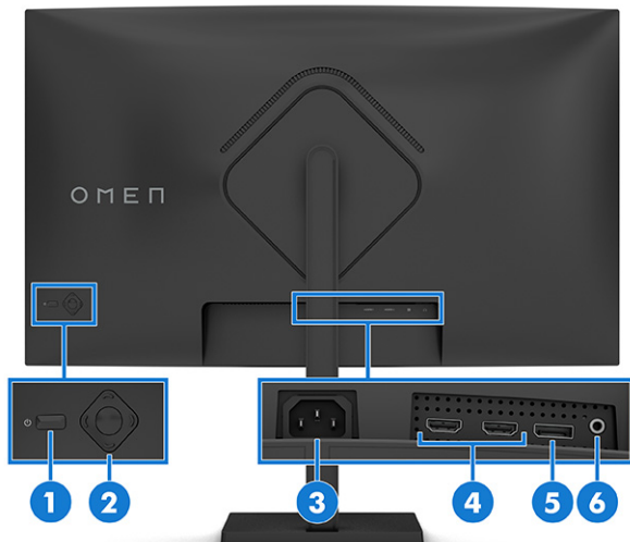
Tabuľka 2-4 Súčasti na zadnej strane a ich popisy
