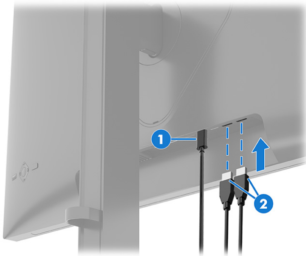
Tabuľka 2-5 Umiestnenia portu USB
