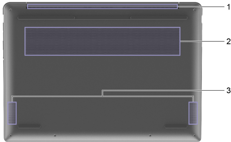
Obrázok 5. Yoga Slim 7 14IMH9—pohľad zospodu
