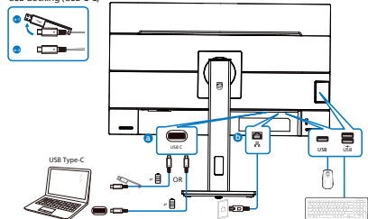
USB docking (USB C-Q)
