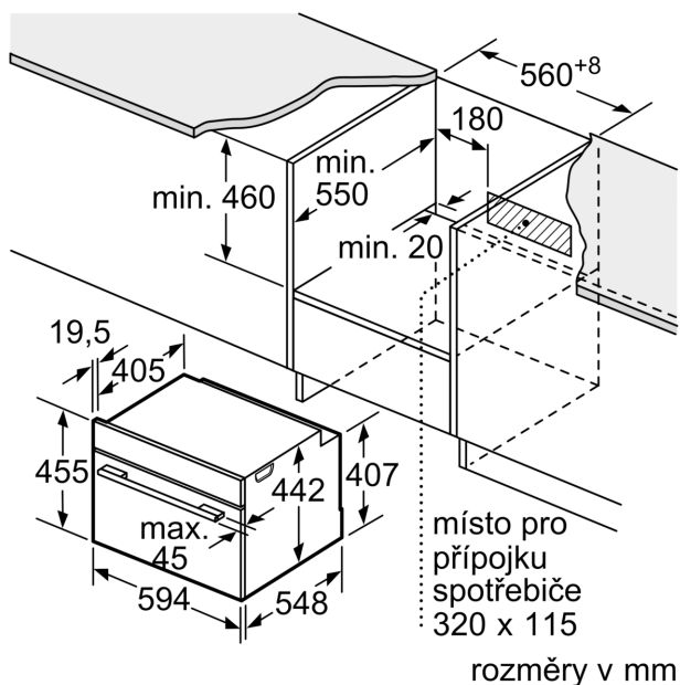
vestavba s varnou deskou
