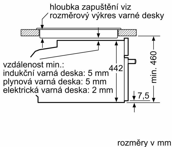
vestavba s varnou deskou
