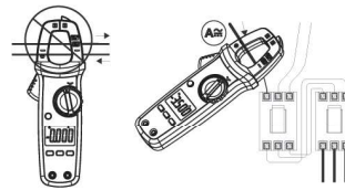
Obrázok 2 - Meranie prúdu
