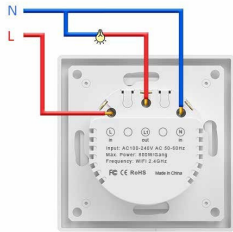
SCHEMA PRIPOJENIA
