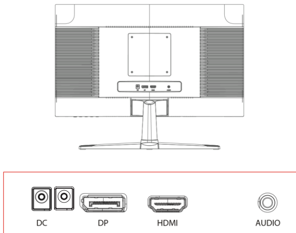
Obrázok 4-1 Vstupné a výstupné rozhranie
