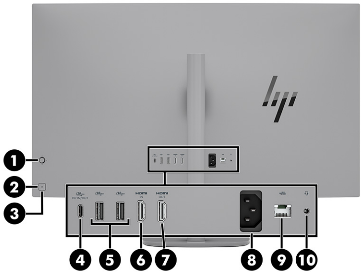
Tabuľka 4-3 Identifikácia súčastí na zadnom paneli
