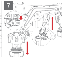
Posuňte tlmič a riadiacu páku do polohy obmedzovača, potom dotiahnite skrutku čeľuste tlmiča
