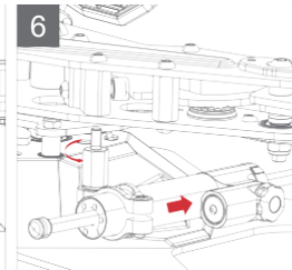
Vložte čeľusť tlmiča a nainštalujte spojenie riadiacej páky
