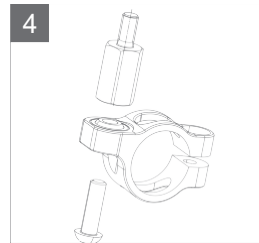
Zmontujte spojenie riadiacej páky s čeľusťou tlmiča
