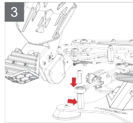
Nainštalujte tlmič
