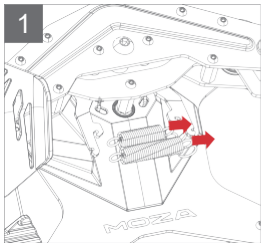
Odstráňte pružiny
