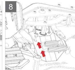
Namontujte znovu pružiny
