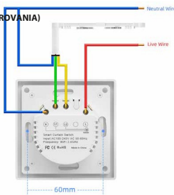
SCHEMA PRÍPOJENIA
