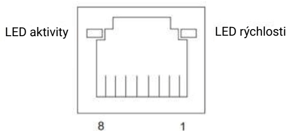
Obrázok 11. Port RJ45 (strana konektora)
