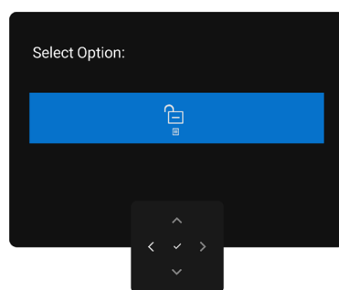
Obrázok 66. Ponuka odomknutia
