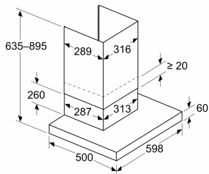
Rozměry v mm Spotřebič v režimu odpadního vzduchu
