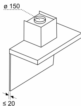
Rozměry v mm Hloubka nástěnného panelu
