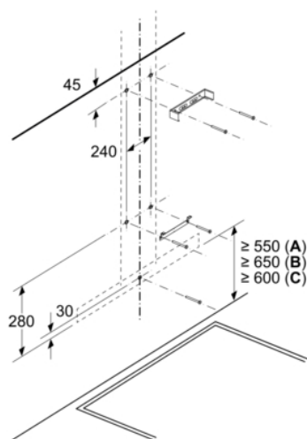
Rozměry v mm Nástěnná instalace s komínem
