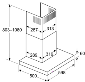
Rozměry v mm Recirkulační systém
